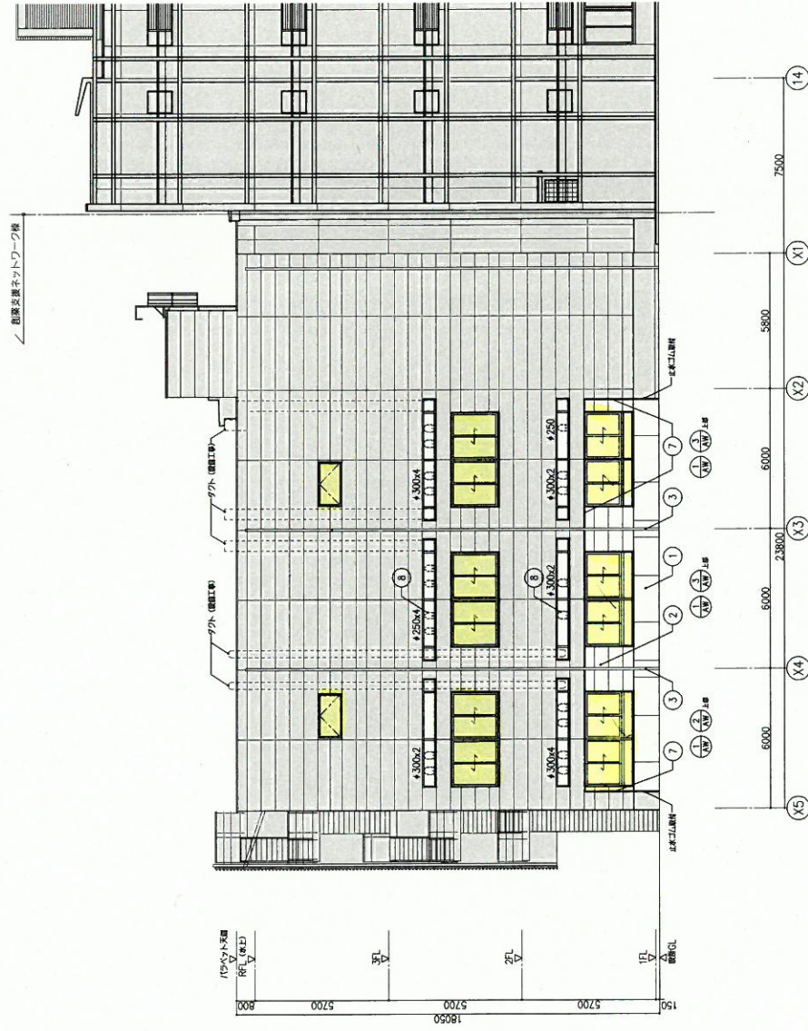
建築・改修 北立面図 1:100
