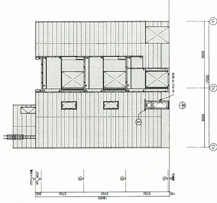
建築・改修 西立面図 1:100
