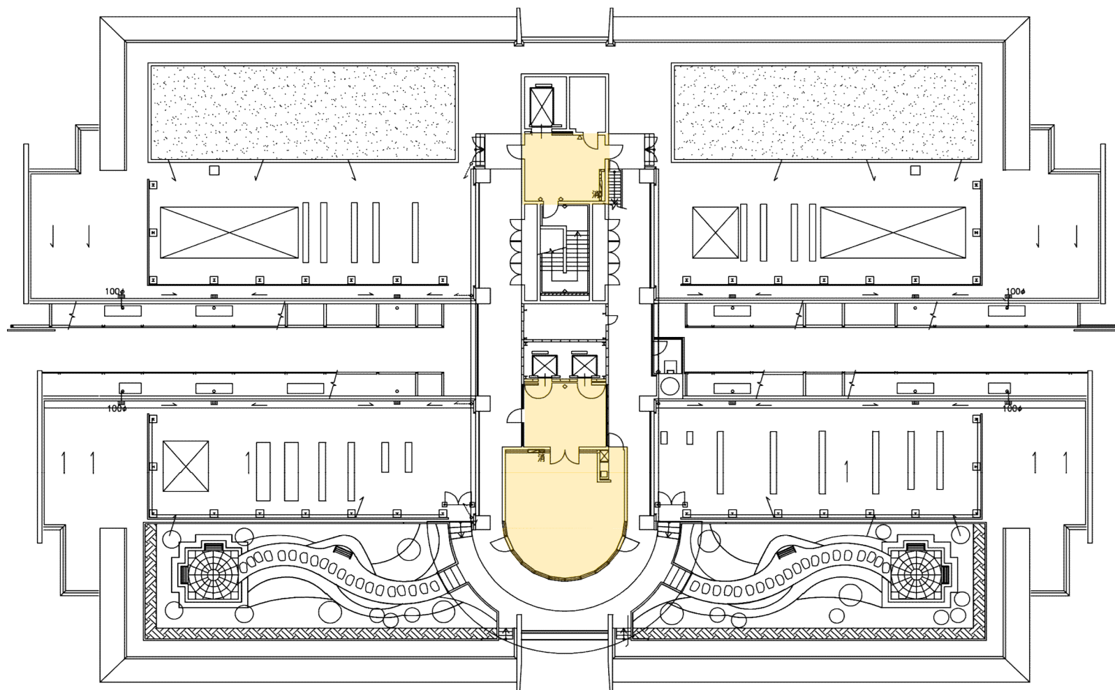
5階平面図
