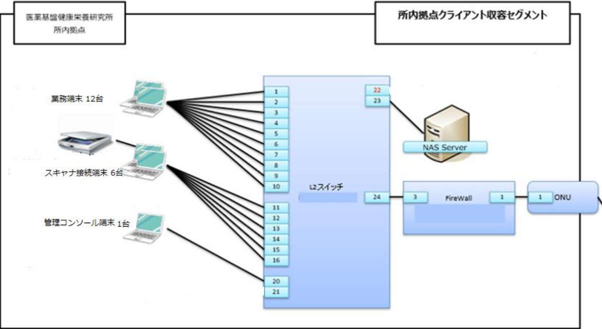
【所内環境 ネットワーク構成】
