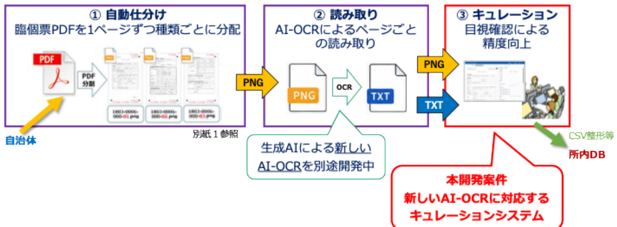
図1 AI-OCR システムの概要
